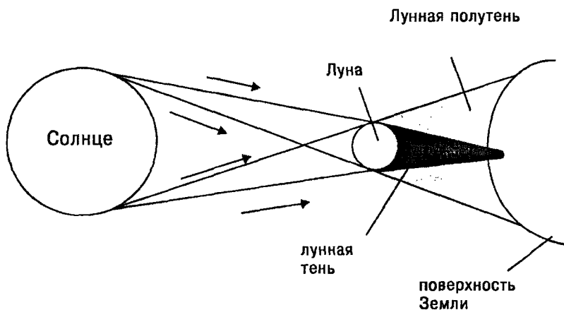
Рис.3.7. Схема солнечного затмения
