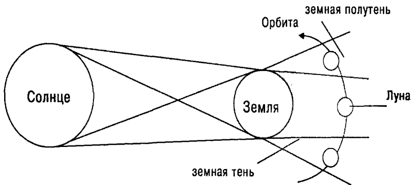
Рис. 3.8. Схема лунного затмения
